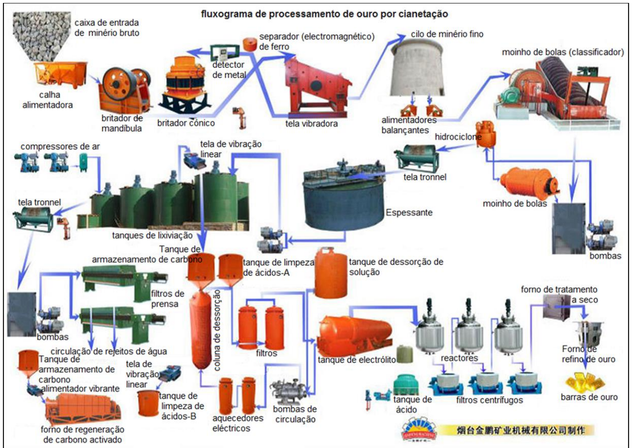
Figura iii. Fluxograma do processamento de ouro
